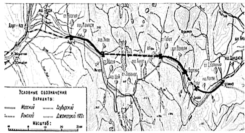
План варианта скоростной железной дороги с нанесением проектной схемы Ленгипротранса 1945–47 гг. (Федоров А.В.)
